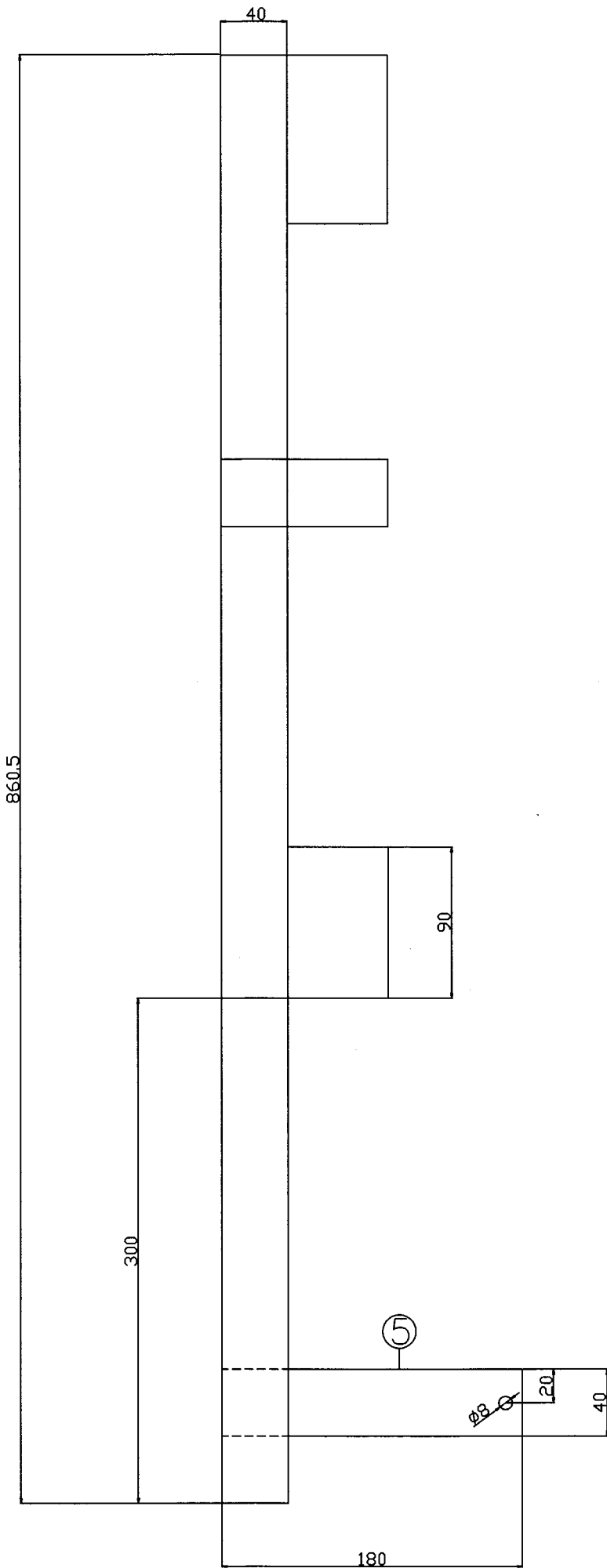
Frame linkerzijaanzicht
